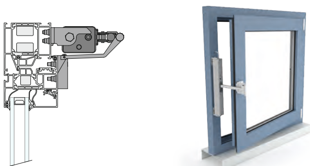
Drehflügelfenster, einwärts öffnend
