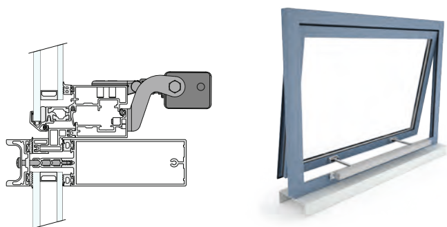
Senk-/Klappfenster, auswärts öffnend
